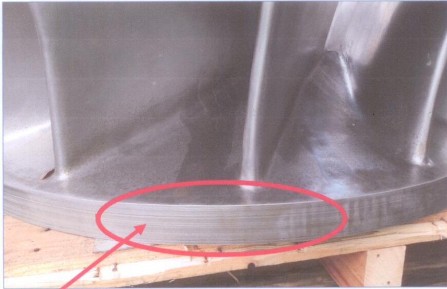
CORONA RODETE DESGASTADA POR LA ARENA, 2 MM DE DESGASTE.
