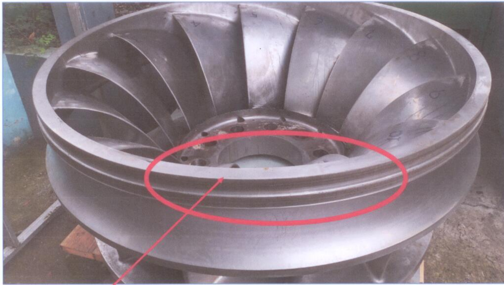
ZONA DE LA BANDA DEL RODETE Y LABERINTO DESGASTADO DE 3 MM DE DESGASTE, DAÑO HECHO POR LA ARENA QUE ESTA ENTRANDO AL TUNEL.
