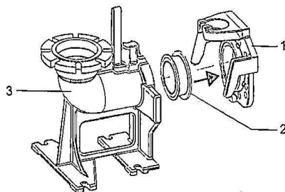
Fig. 25 Pedestal en arco (versión básica sólo ME4) DN 100/150/200
