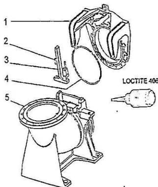
Fig. 26 Pedestal ecodado DN 100 - 500
