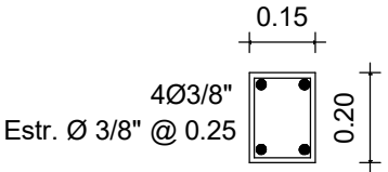
VIGA DE AMARRE NIVEL DE PISO Y TECHO
