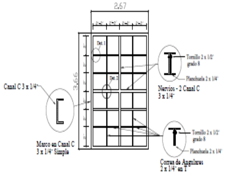
Esquema Reforzado de los Paños 1 al 6
