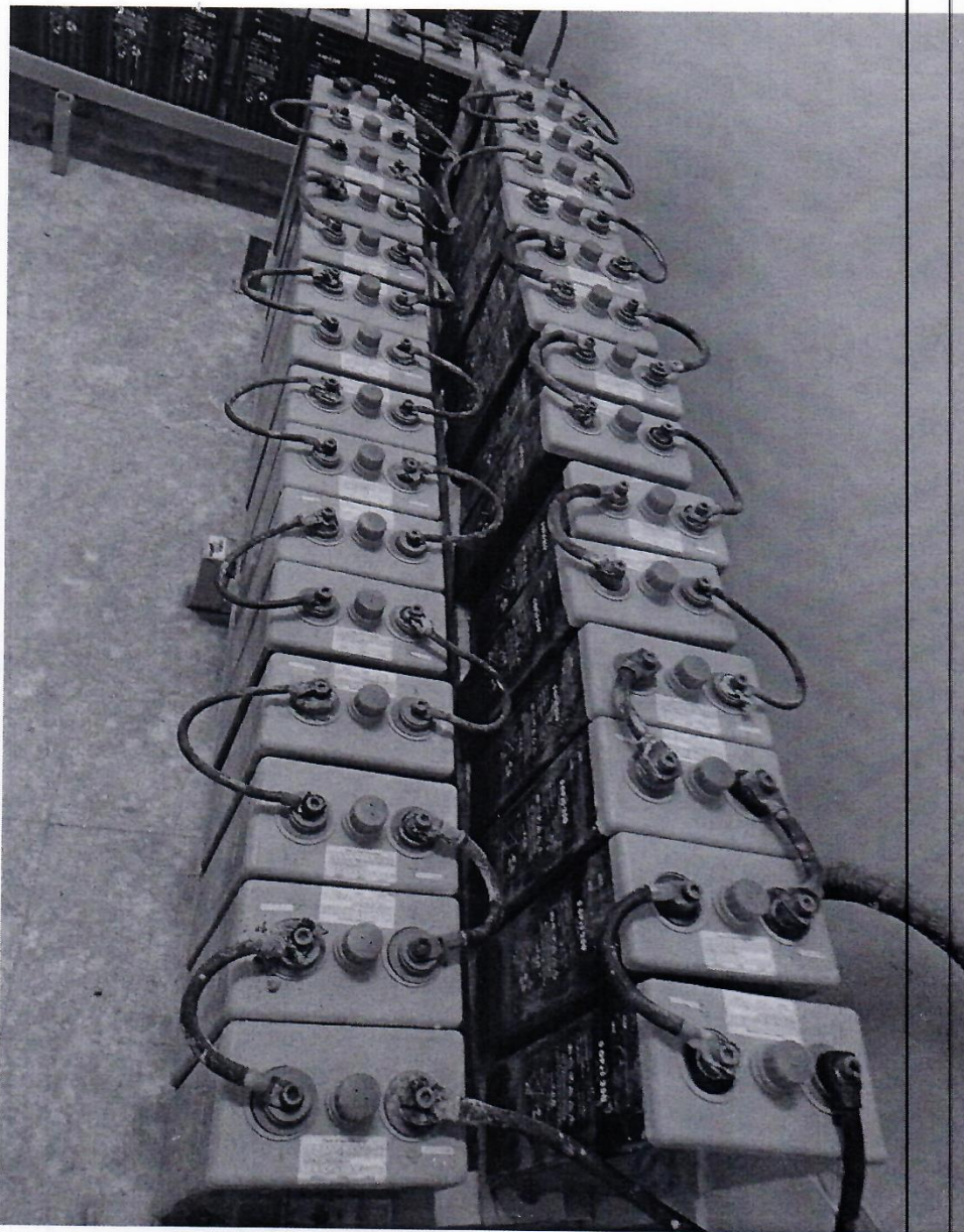
BANCO DE BATERIAS CENTRAL DOMINGO RODRIGUEZ
