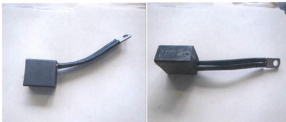
Imágenes correspondientes a las Escobillas de Grafito de dimensiones: 40 x 25 x 50 mm, antes solicitadas.
