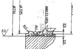
DETALLE 1 - ECH:1 DETALLE 1 - ESCALA:1
