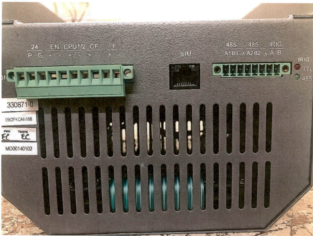
Alimentación y conexiones del CPXCAN
