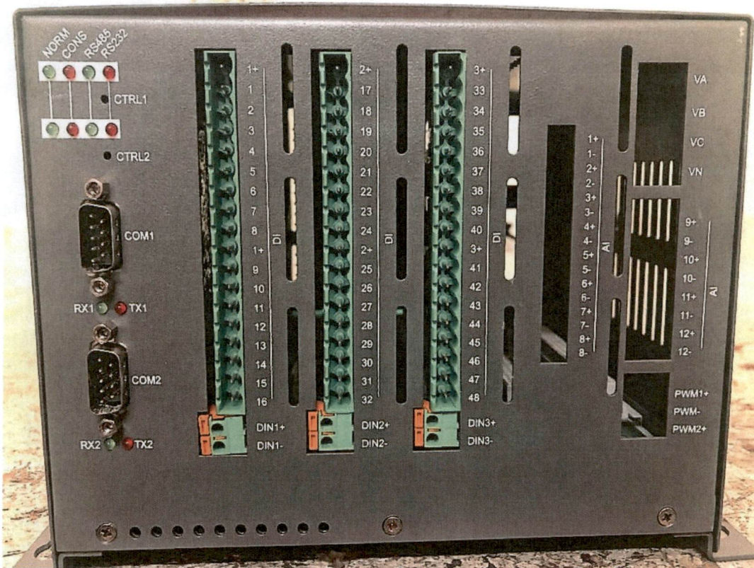
Alimentación y conexiones del Multican
