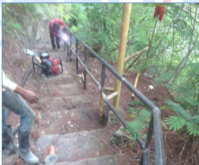
Instalación de barandas escalera presa de Jimenoa, Campamento Jimenoa.
