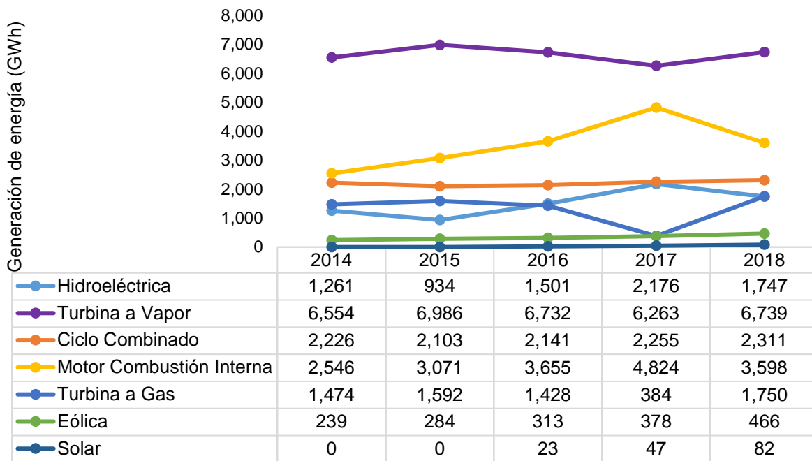
Gráfico Anexo I. 3 Cantidad de generación de energía (GWh) por tipo de tecnología (6)
